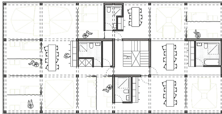
Grundriss 1. Obergeschoss | Bauphase 02
